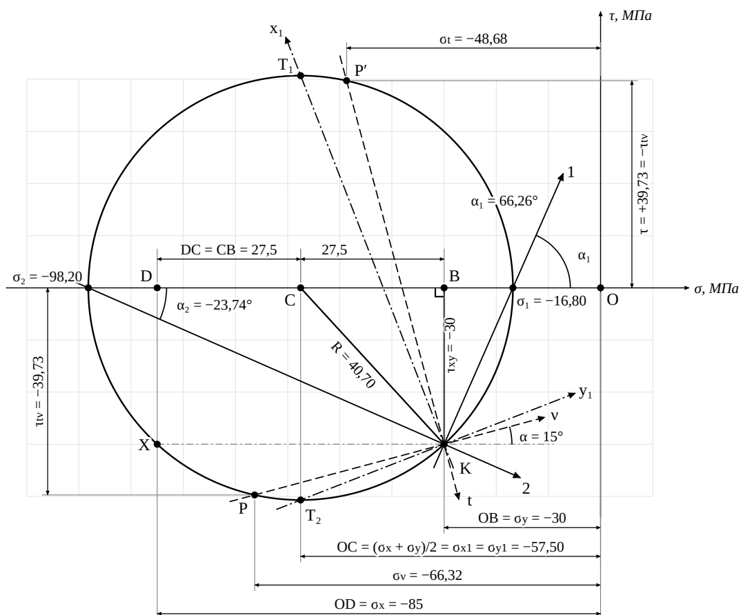
Рис. 7 — круг Мора, 1 см = 10 МПа (сетка — 10 МПа). Прямые из полюса К: 1 и 2 — главные направления; x_1 и y_1 — оси площадок экстремальных касательных напряжений (через T_1, T_2 ); v и t — площадки под 15^\circ и 105^\circ (через P, P' ). Координаты P и P' показаны размерами \sigma_v, \tau_v, \sigma_t .
